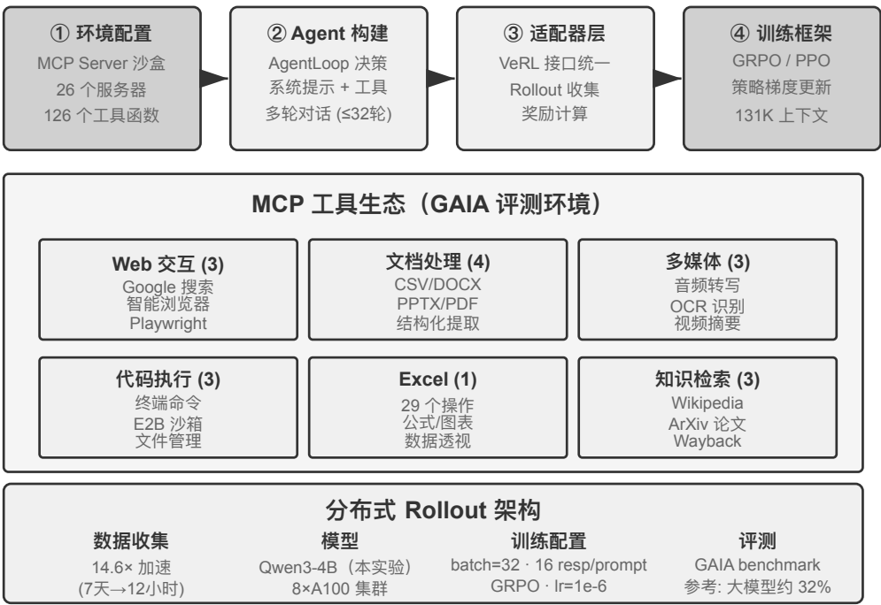
图 7-18 AWorld-train MCP 沙盒训练架构与工具生态
