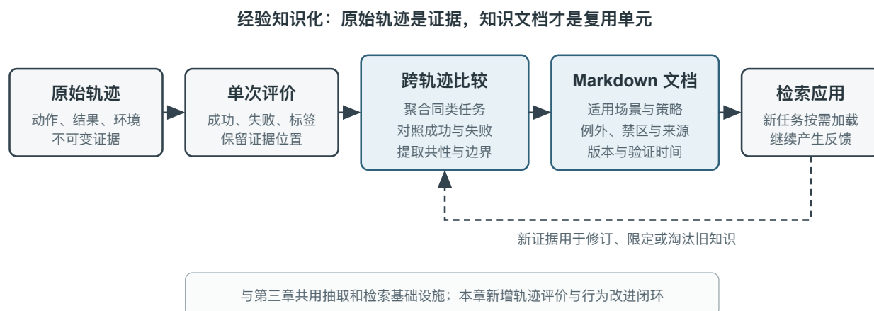
图 8-4 从已评价轨迹到经验知识文档
