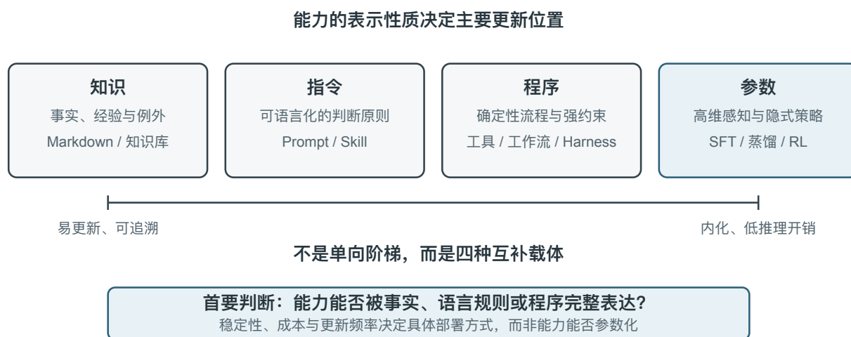
图 8-3 持续进化的四种更新方式
