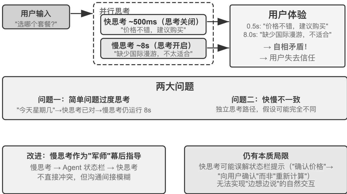
图 9-5 快/慢思考架构与方案对比
