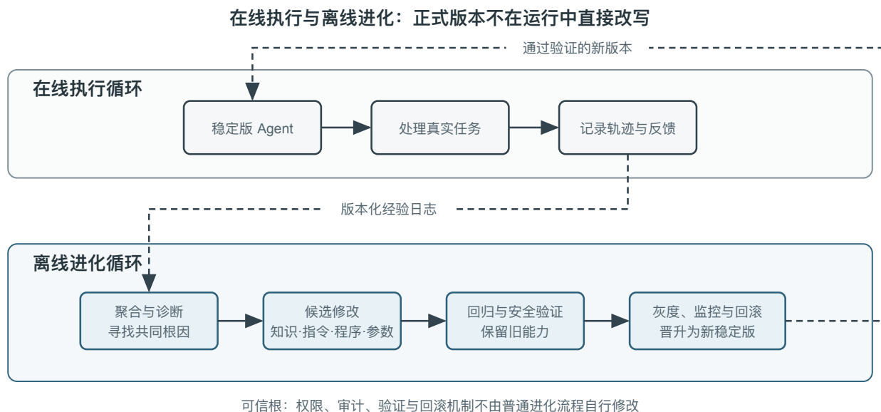
图 8-5 在线执行与离线进化的双循环
