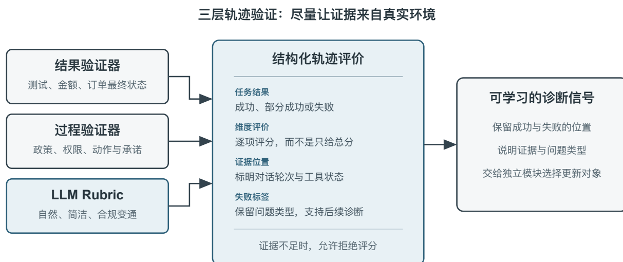
图 8-2 从环境结果到 LLM Rubric 的三层轨迹验证
