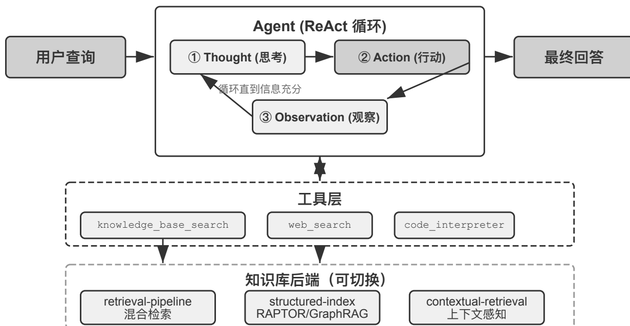
图 3-13 智能体化 RAG 系统架构
