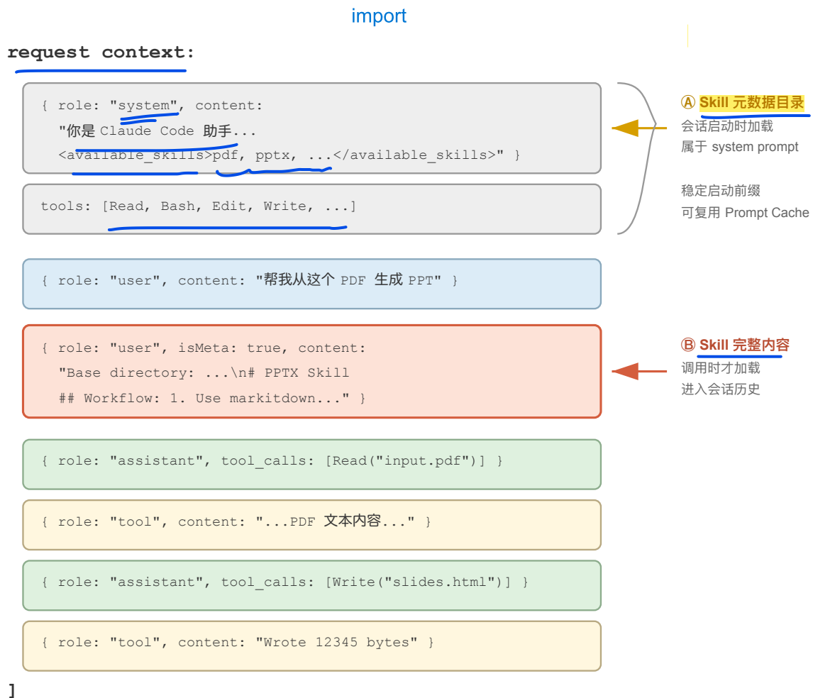
图 2-12 启用 Skills 后 Agent Trajectory 的完整结构
