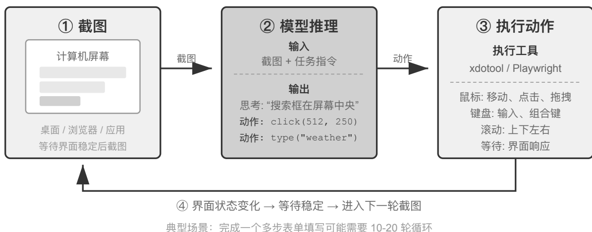
图 9-7 Computer Use Agent 的感知-思考-行动循环
