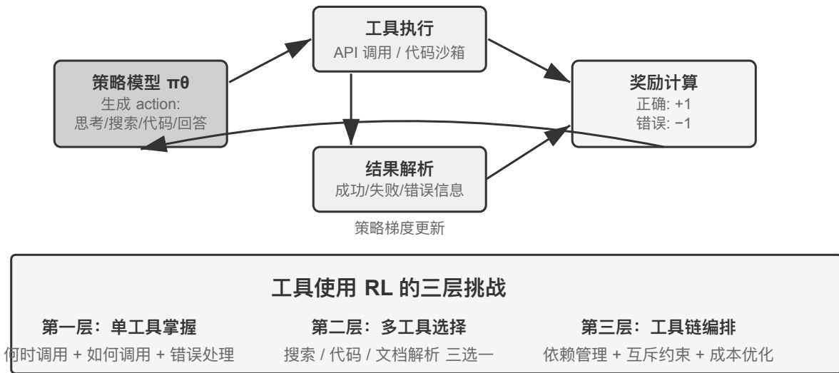
图 7-16 工具调用 RL 奖励循环
