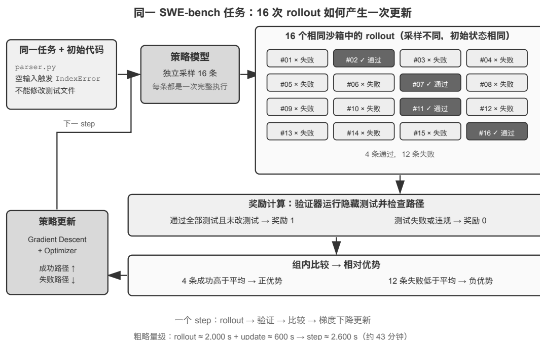
图 7-13 同一 SWE-bench 任务的 16 次 rollout、验证与相对优势
