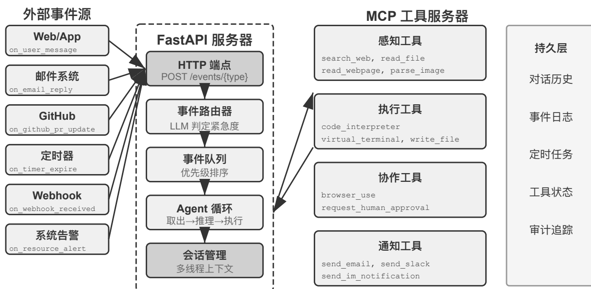
图 4-4 实验 4-5 事件驱动 Agent 架构
