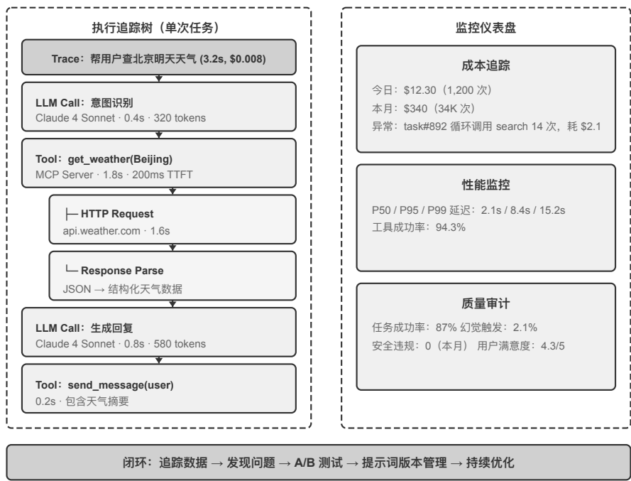
图 6-6 可观测性技术栈
