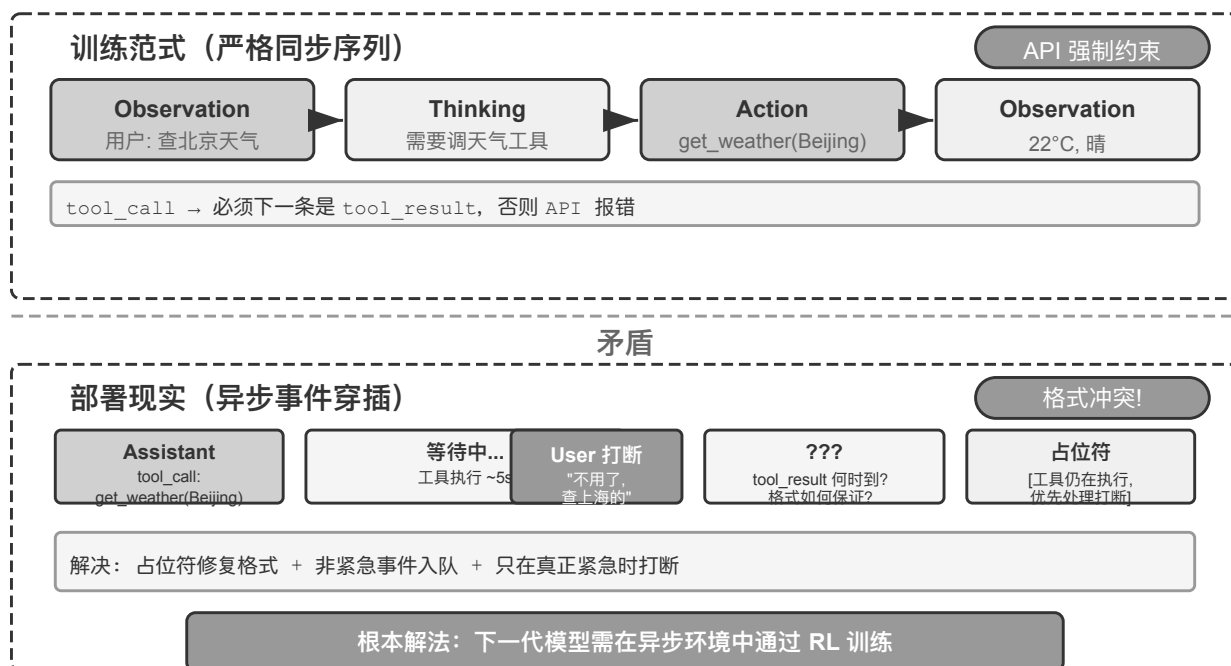
图 4-5 同步训练范式与异步部署现实
