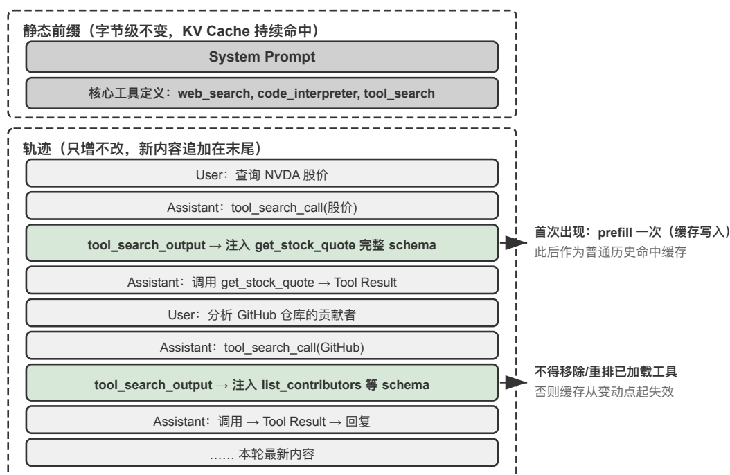
图 4-9 动态发现后的上下文结构：工具 schema 散落在轨迹各处
