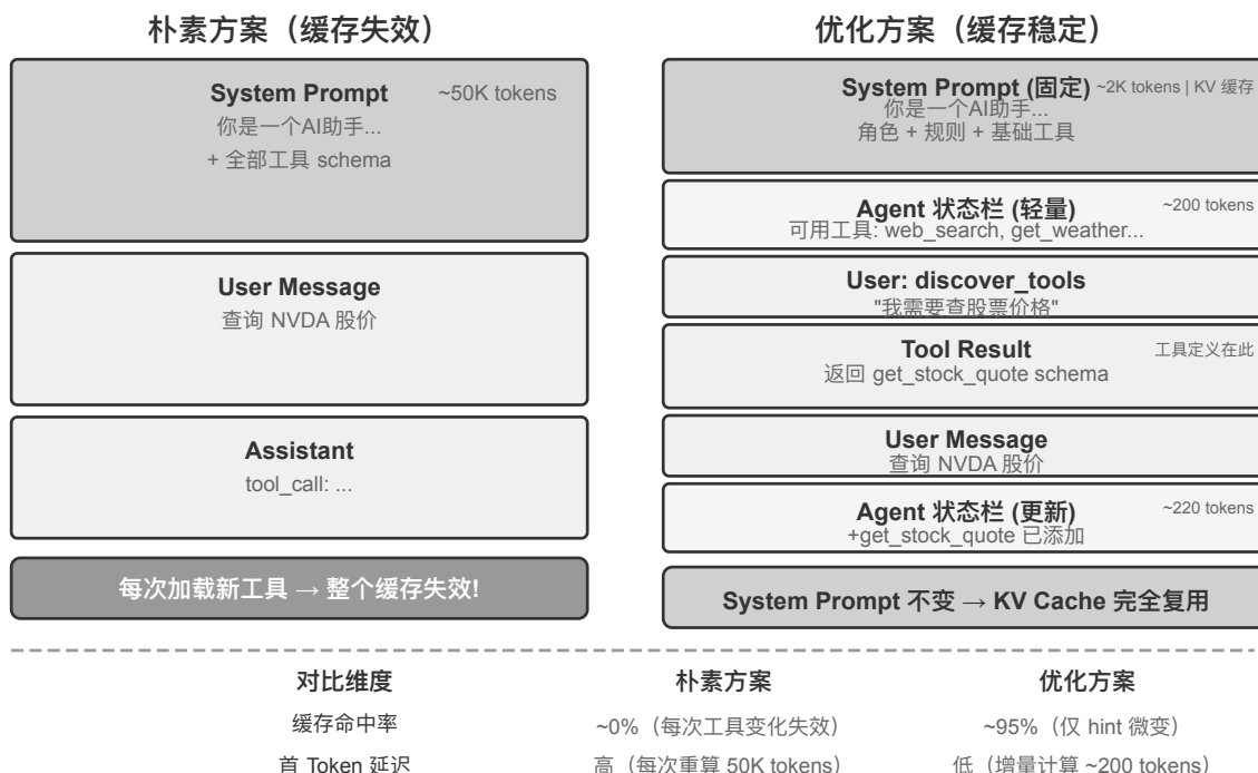
图 4-8 工具动态加载的 KV Cache 优化
