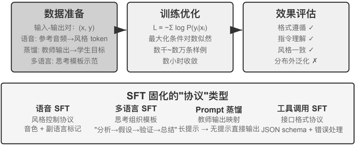
图 7-10 监督微调（SFT）流水线
