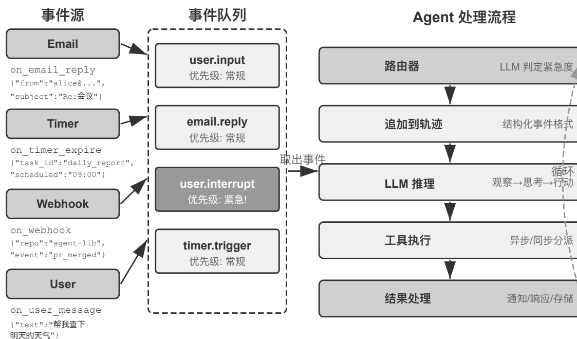
图 4-2 事件驱动的异步 Agent 架构
