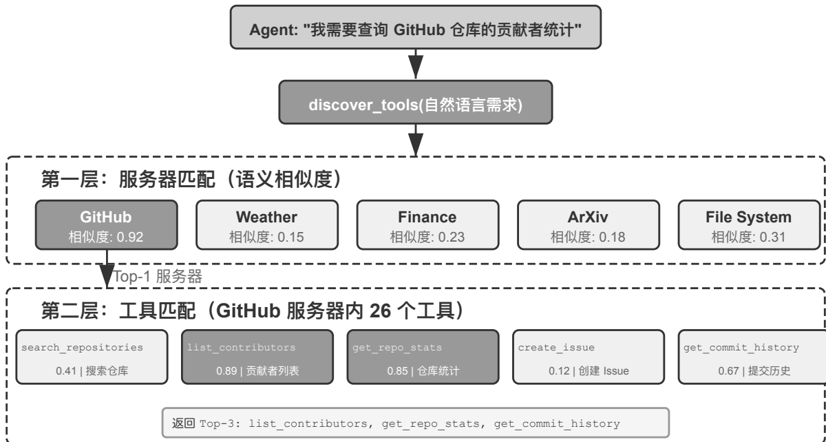
图 4-7 层次化工具匹配（服务器级 → 工具级两层语义搜索）
