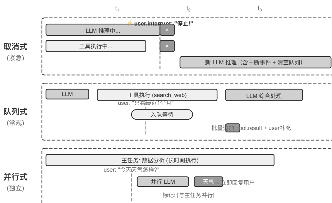
图 4-3 异步事件处理的三种策略
