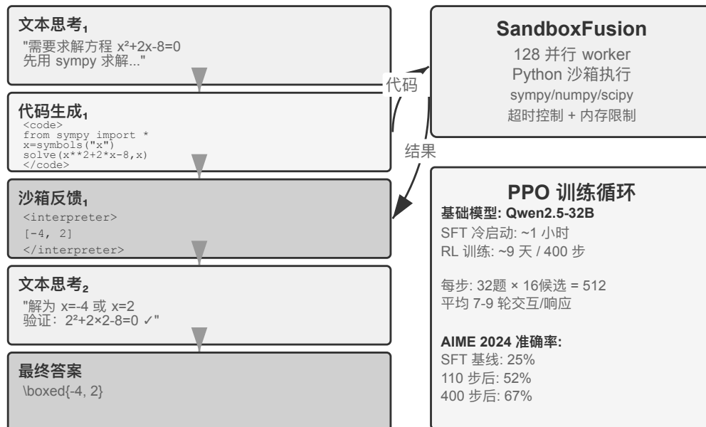
图 7-17 ReTool 交织文本-代码思考与沙盒执行反馈循环
