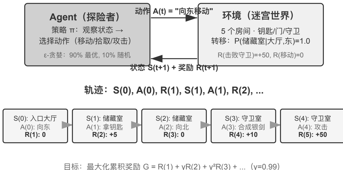
图 7-1 强化学习 Agent-环境交互循环
