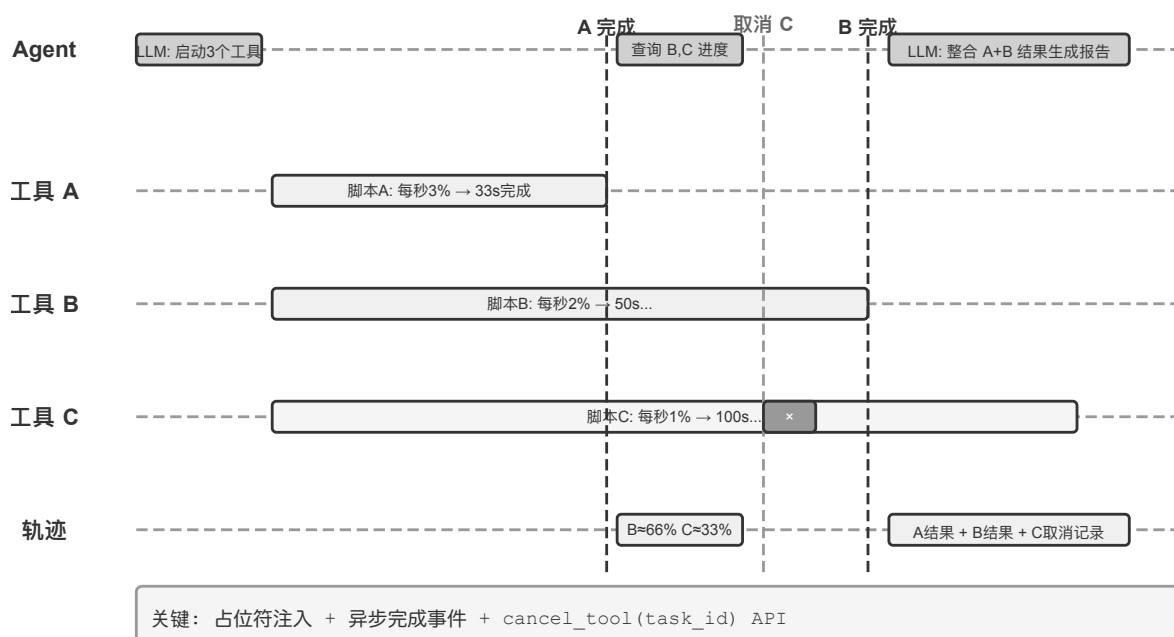
图 4-6 实验 4-6 异步 Agent 打断与恢复
