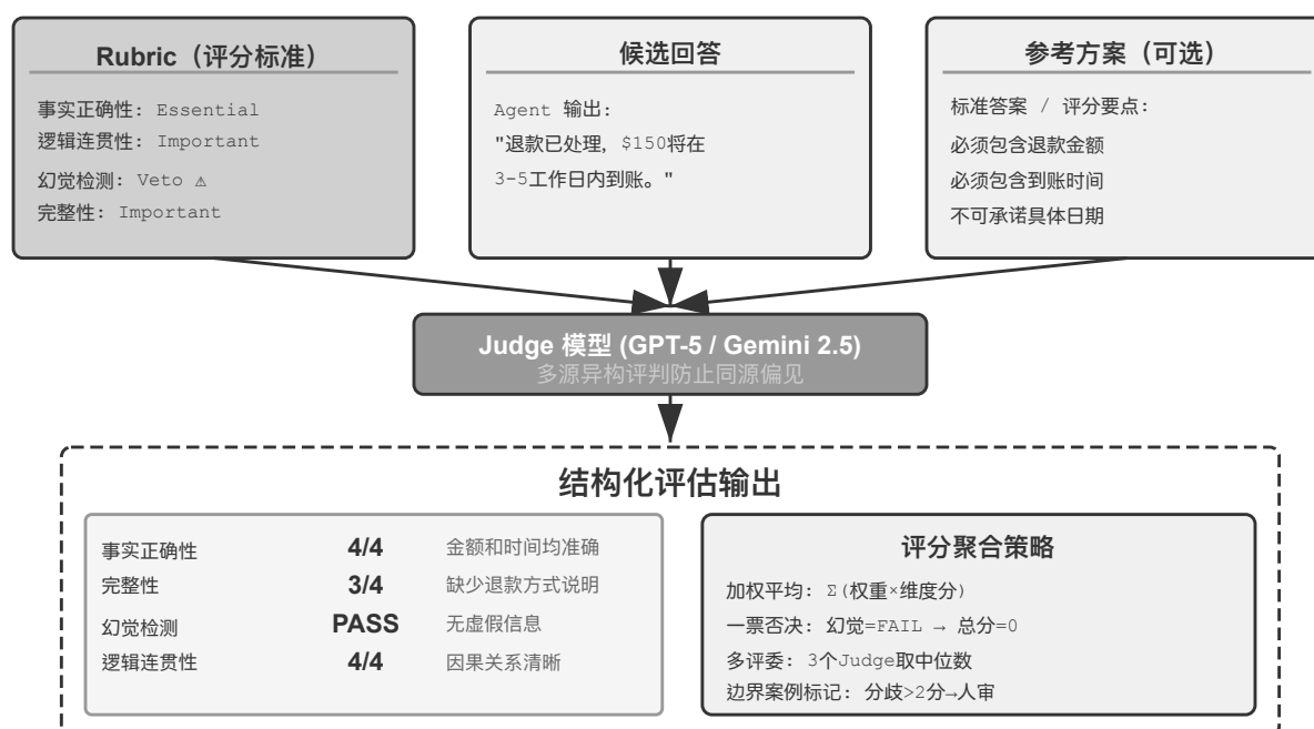
图 6-4 LLM-as-a-Judge 流水线
